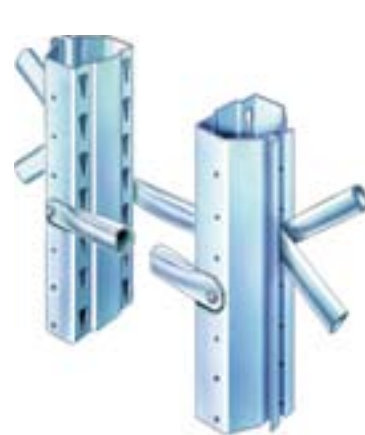
Conjunto distanciador de 300 mm para hilera doble con fijaciones.
